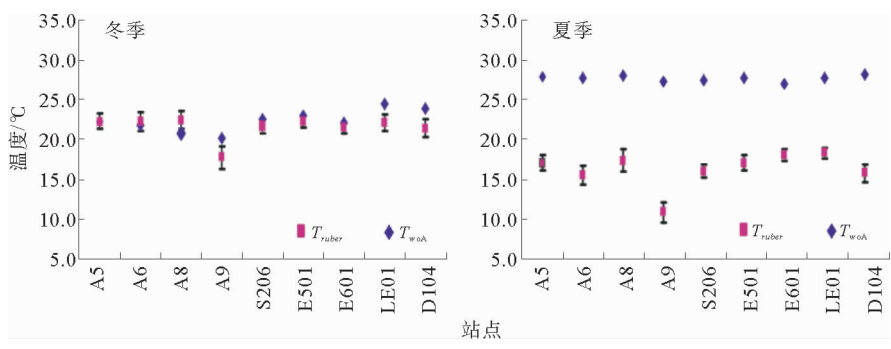
图 3 南海北部各站点 T_{ruber} 与 T_{WOA} 的比较
