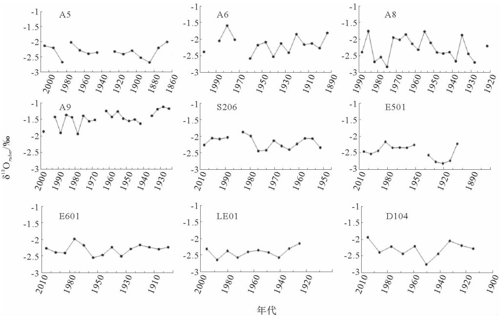
图 2 南海北部 9 个钻孔有孔虫壳体氧同位素测试结果(V-PDB) Fig. 2 The \delta^{18}\text{O}_{ruber} values of each sediment core (V-PDB)
